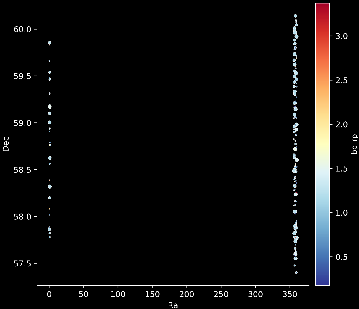
APOGEE DR17 Field: [CVZTILE_088+35_btx] Stars: 181
