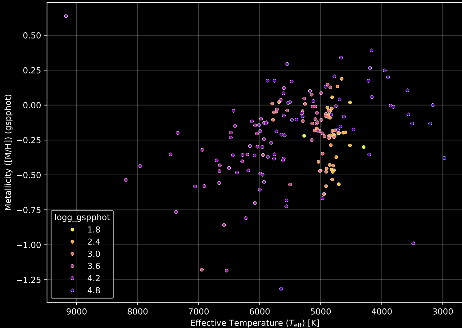
APOGEE DR17 Field: [CVZTILE_088+35_btx] Stellar Population Parameters (n= 181)
