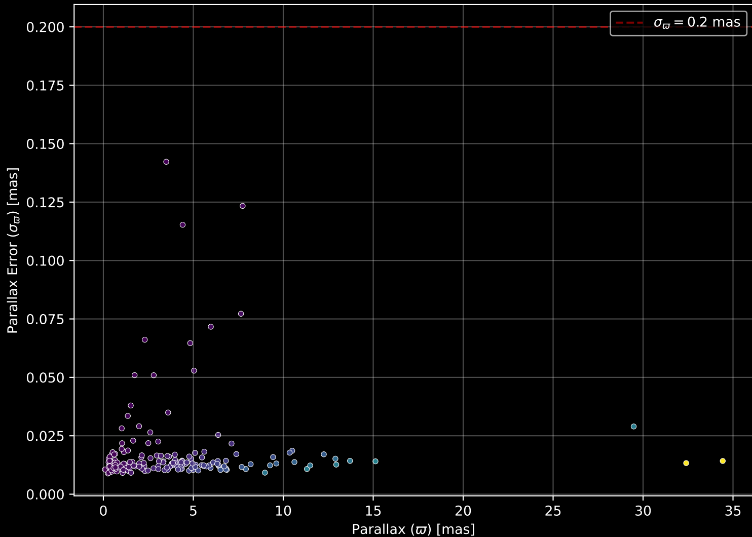
APOGEE DR17 Field: [CVZTILE_088+35_btx] Parallax Quality (n= 181)
